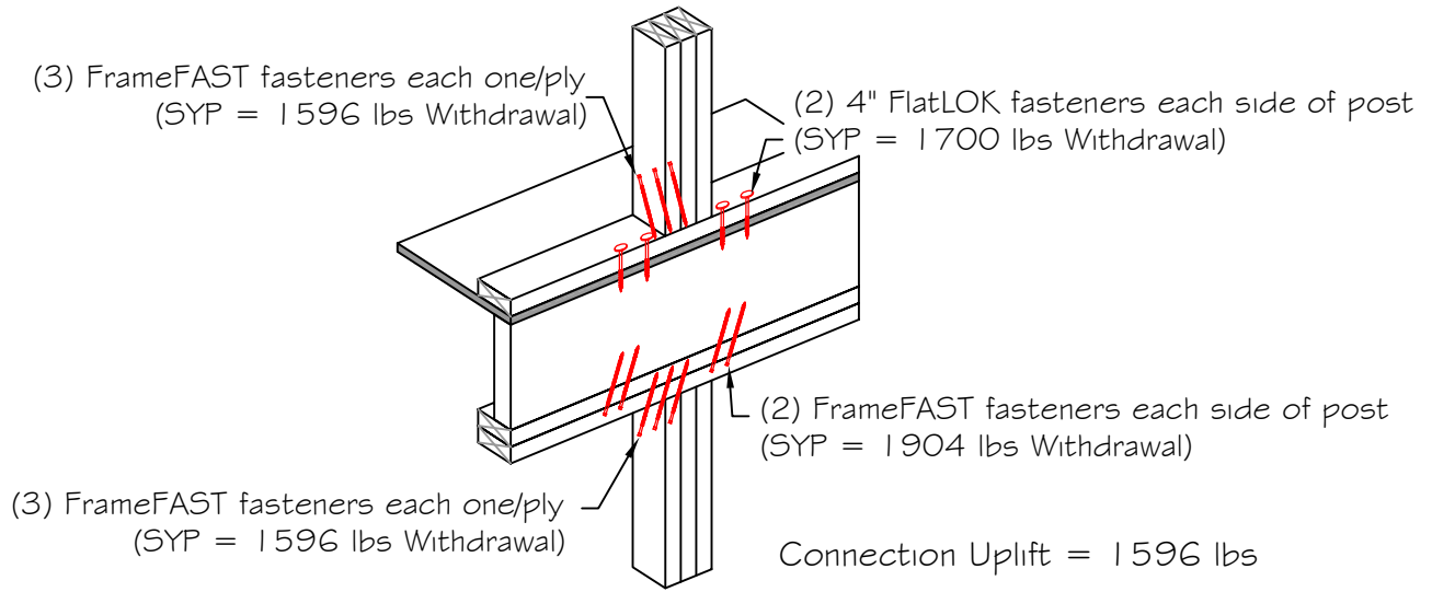
Triple Stud Pack - Isometric
